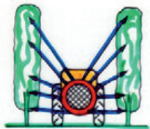
Sprühgerät mit Radialgebläse
